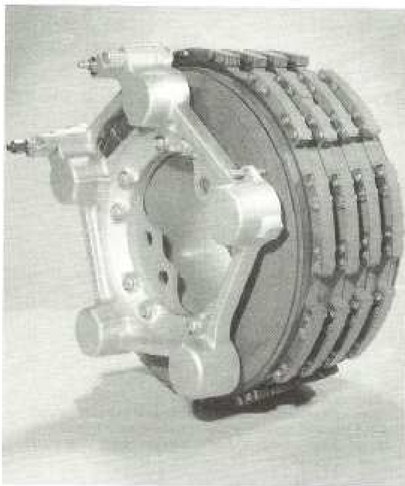
Paquete de frenos. Observe los cinco pistones hidráulicos y los discos de freno. (Falta Dunlop)
