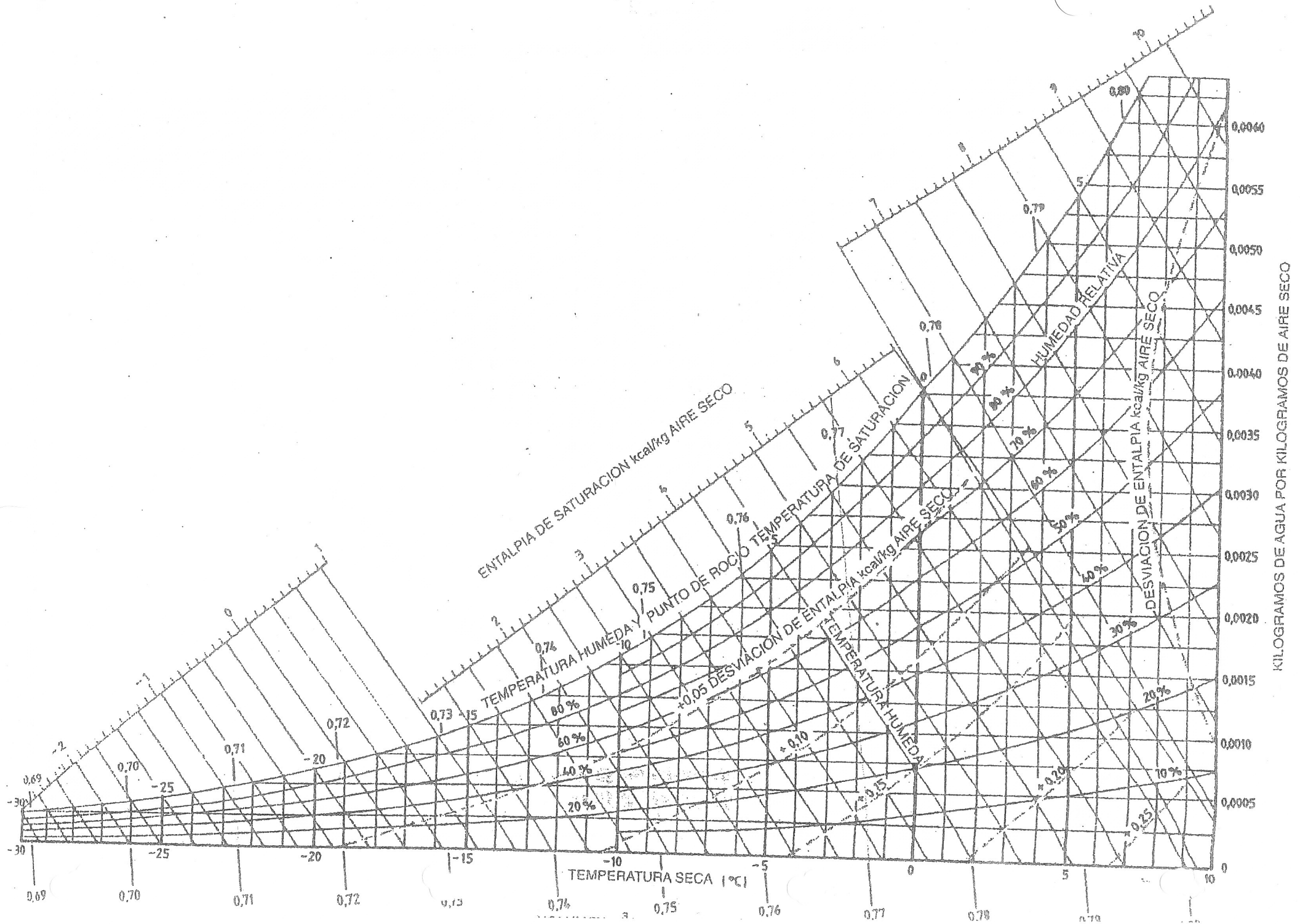
Figura 8. Diagrama psicrométrico del aire a bajas temperaturas.
